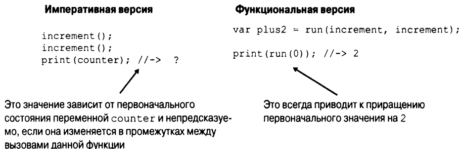
Рис. 1.2. Сравнение функциональной и императивной версий функции increment() . Результат выполнения императивной версии непредсказуем и может быть непостоянным, поскольку внешняя переменная counter способна измениться в любой момент, нарушив результат последующих вызовов данной функции. А ссылочно-прозрачная функциональная версия всегда эквивалентно корректна и не оставляет места для ошибок
