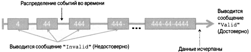
Рис. 8.13. Наглядное представление событий, наступающих в связи с обновлением номера социального страхования учащегося, в виде наблюдаемого потока, создаваемого в результате подписки на событие типа change в поле ввода этого номера
