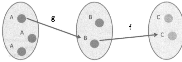
Рис. 4.10. Наглядная демонстрация преобразования типов входных и выходных данных в функциях g и f . В частности, функция g преобразует значения типа A в значения типа B , а функция f — значения типа B в значения типа C . Композиция происходит потому, что функции f и g совместимы по типам
