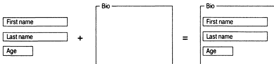
Рис. 4.7. Объединение трех простых виджетов ввода текста с виджетом контейнера для создания компонента биографической формы
