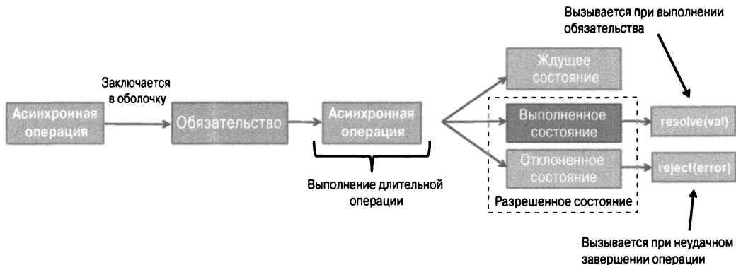
Рис. 8.5. Порядок заключения операции в оболочку монады типа Promise и предоставления двух обратных вызовов: одного — для выполнения функции resolve() , а другого — для выполнения функции reject() . Вначале обязательство находится в ждущем состоянии, а затем переходит в выполненное или отклоненное состояние. Для этого вызываются функции resolve() или reject() соответственно, после чего обязательство переходит в разрешенное состояние
