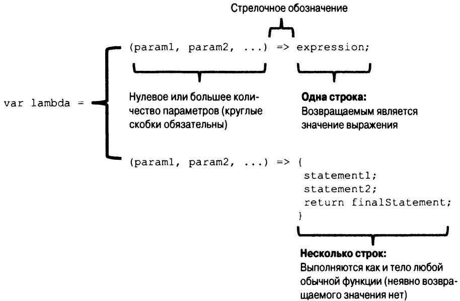
Рис. 3.3. Разбор структуры стрелочных функций. В правой части лямбда-выражения указывается единственное выражение или ряд операторов, заключаемых в фигурные скобки
