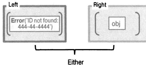
Рис. 5.9. В структуре типа Either можно хранить объект (справа) или ошибку типа Error с соответствующей информацией из трассировки стека (слева). Это удобно, если требуется предоставить единственное возвращаемое значение, которое может также содержать сообщение об ошибке на случай сбоя
