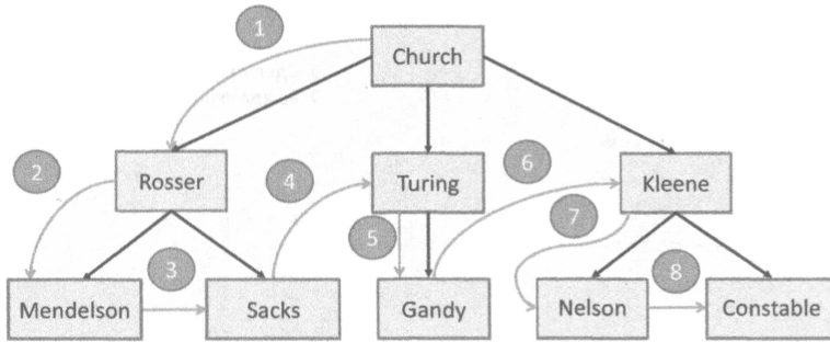
Рис. 3.9. Рекурсивный характер обхода дерева в ширину начинается с корневого узла и продолжается сначала влево, а затем вправо
