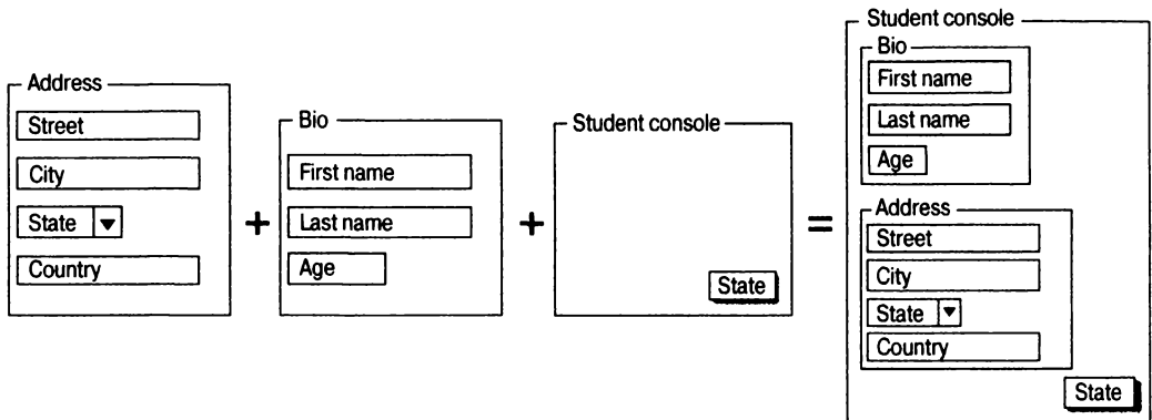
Рис. 4.8. Виджет консольной формы для заполнения сведений об учащемся, созданной из адресной и биографической форм, кнопки и контейнера
