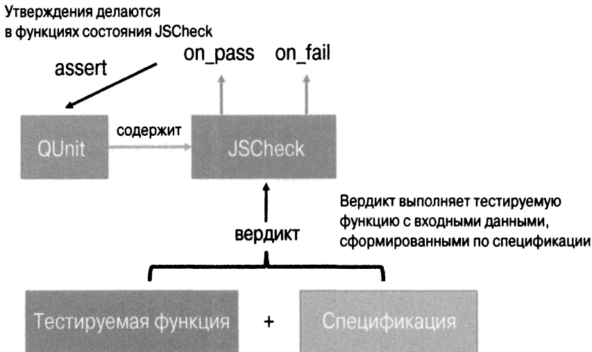
Рис. 6.8. Интеграция главных компонентов JSCheck и QUnit для тестирования на основе свойств. Тест QUnit инкапсулирует спецификацию теста JSCheck. Спецификация и тестируемая функция предоставляются функции verdict() , которая интерпретируется в JSCheck для выполнения обратных вызовов, когда тесты проходят или не проходят. Эти обратные вызовы могут быть использованы для инициирования утверждений в модульных тестах QUnit
