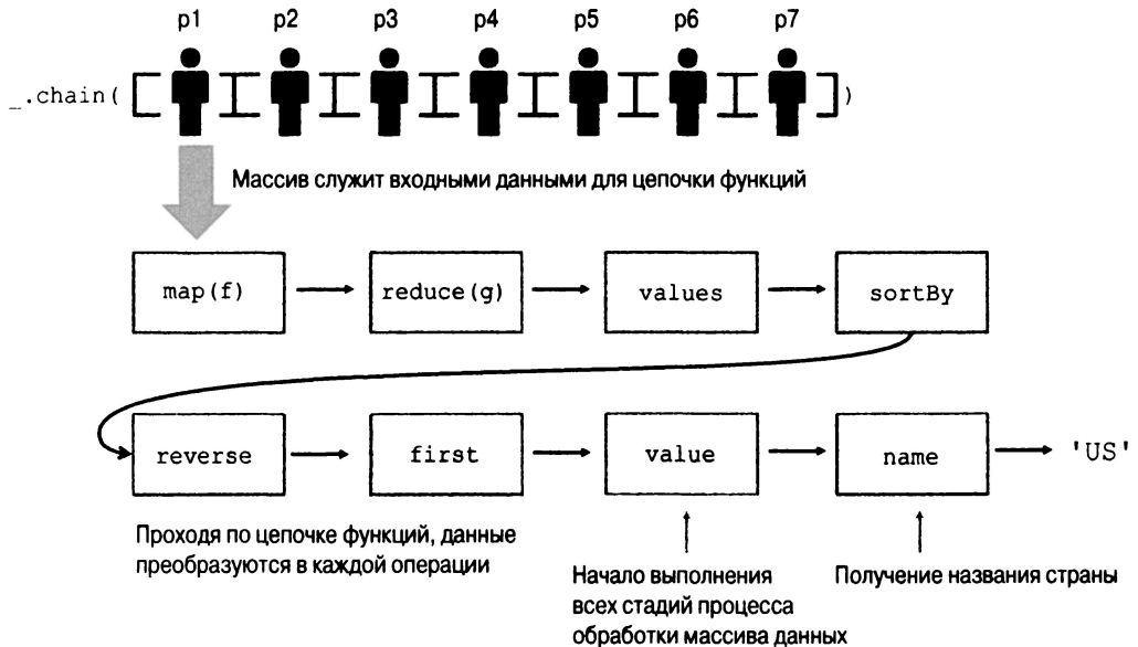
Рис. 3.7. Поток управления программой, составленной из цепочек функций библиотеки Lodash. Массив объектов типа Person обрабатывается в ходе выполнения последовательного ряда операций, проходя через которые данные в конечном итоге сводятся к единственному значению
