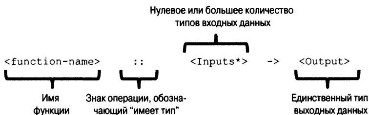
Рис. 4.1. Принятое в языке Haskell обозначение функции при ее определении. В этом обозначении описывается имя функции, после которого следует операция, задающая типы входных и выходных данных этой функции
