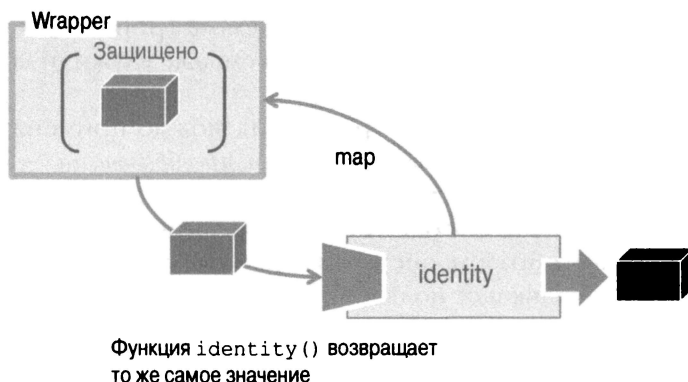
Рис. 5.2. Операция map служит для безопасного доступа к объекту типа Wrapper и манипулирования заключенными в него значениями. В данном случае операция преобразования ( map ) применяет функцию тождественности ( identity ) к оболочке, чтобы извлечь из нее значение как из контейнера
