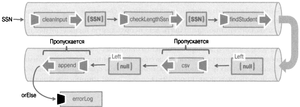
Рис. 5.13. Поэтапный поток выполнения той же самой программы при неудачном завершении функции findStudent() , что оказывает влияние на остальную часть композиции. Независимо от характера сбоя в любом месте конвейера, программа остается отказоустойчивой, корректно пропуская любые процедуры, зависящие от данных
