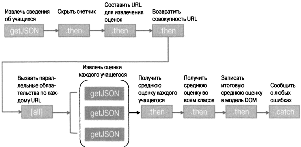
Рис. 8.8. Продвижение поведения через линейно соединяемые и параллельно используемые обязательства с помощью метода Promise.all() . В каждом блоке с методом then() содержится функция, преобразующая передаваемые ей данные. Эффективность данного кода объясняется тем, что в нем порождается несколько параллельных соединений для одновременного извлечения всех данных
