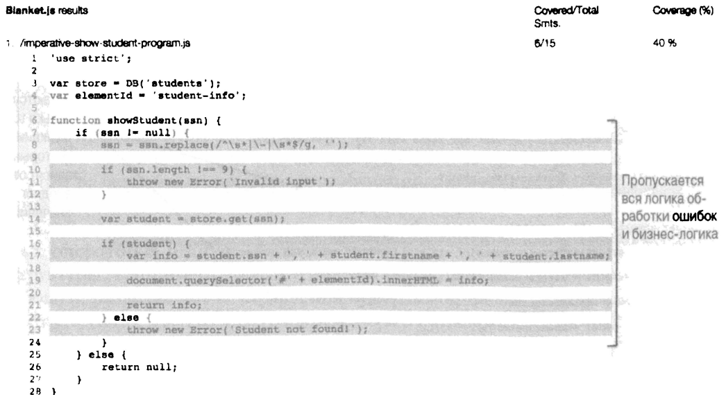
Рис. 6.12. При тестировании императивной версии программы showStudent пропускается положительный путь ее выполнения. В итоге выполняется лишь несколько строк кода, а его покрытие тестами составляет всего 40%
