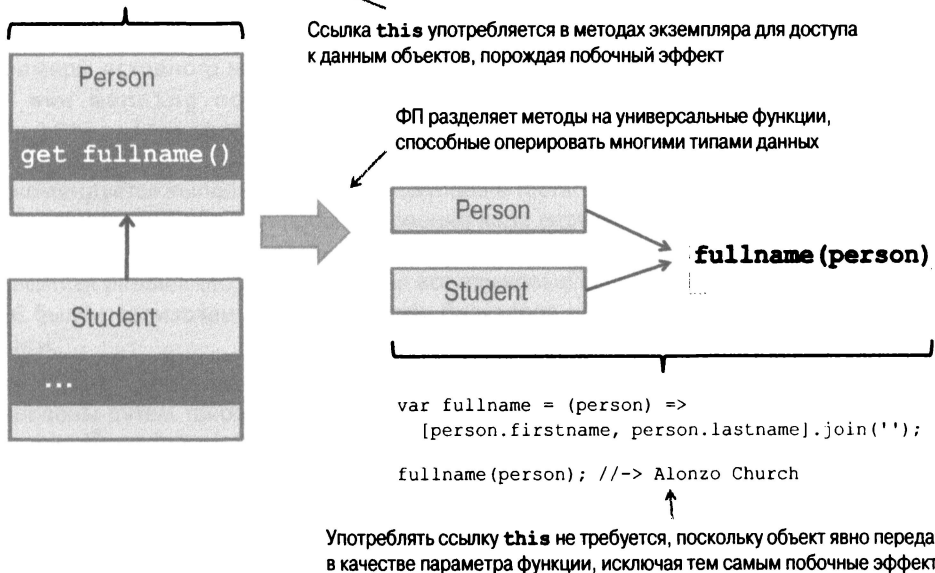
Рис. 2.2. ООП сосредоточено на создании иерархий наследования (например, типа Student от типа Person ) с методами и тесно связанными вместе данными, а ФП — на создании универсальных полиморфных функций, оперирующих разными типами данных, исключая применение ссылки this
