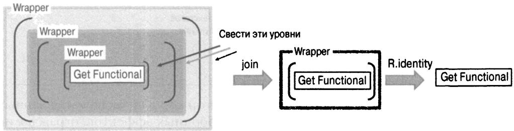
Рис. 5.7. Рекурсивное сведение вложенной монадической структуры с помощью функции join() подобно очистке лука от шелухи
