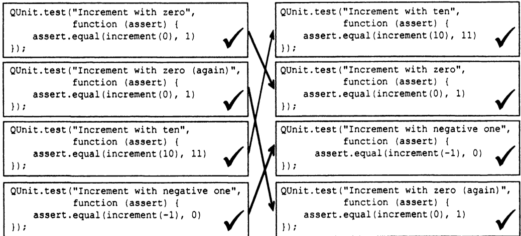
Рис. 6.5. Тесты функциональной версии функции increment() можно повторять и выполнять в любом порядке, неизменно получая одинаковые результаты
