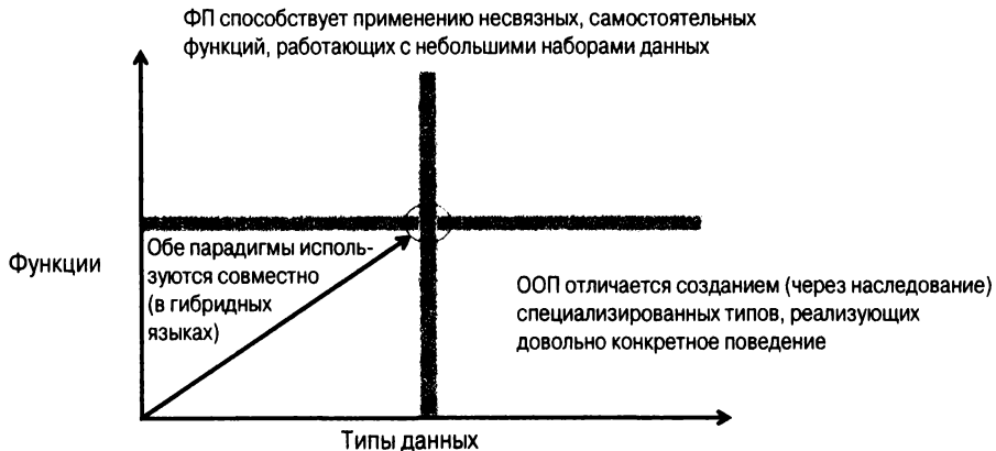
Рис. 2.1. ООП способствует установлению логической связи многих типов данных со специализированным поведением, тогда как ФП сосредоточено на связывании операций с этими типами данных через композицию. Имеется удобное место, где обе парадигмы программирования могут использоваться продуктивно. И это вполне возможно в таких гибридных языках, как Scala , F# и JavaScript
