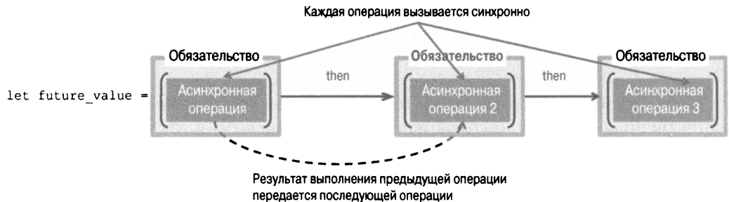
Рис. 8.6. Последовательность обязательств, связанных в цепочку через метод then() . Каждый вызов метода then() производится последовательно с одним обещанным значением после другого, как только будет выполнено каждое обязательство
