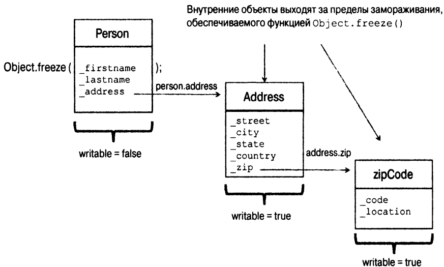
Рис. 2.3. Несмотря на то что объект типа Person заморожен, его внутренние свойства (например, _address ) не были заморожены. Таким образом, вложенное свойство person.address.country подвержено изменениям. Такое замораживание оказывается мелким, поскольку заморожены только свойства верхнего уровня иерархии
