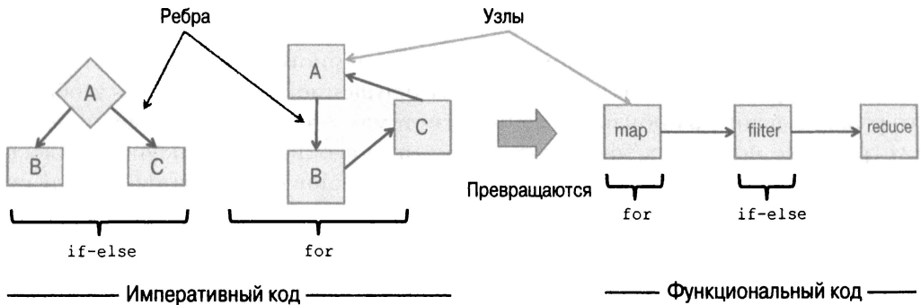
Рис. 6.15. Императивные блоки условных операторов if-else и циклы for в императивном коде превращаются в операции map , filter и reduce в функциональном коде
