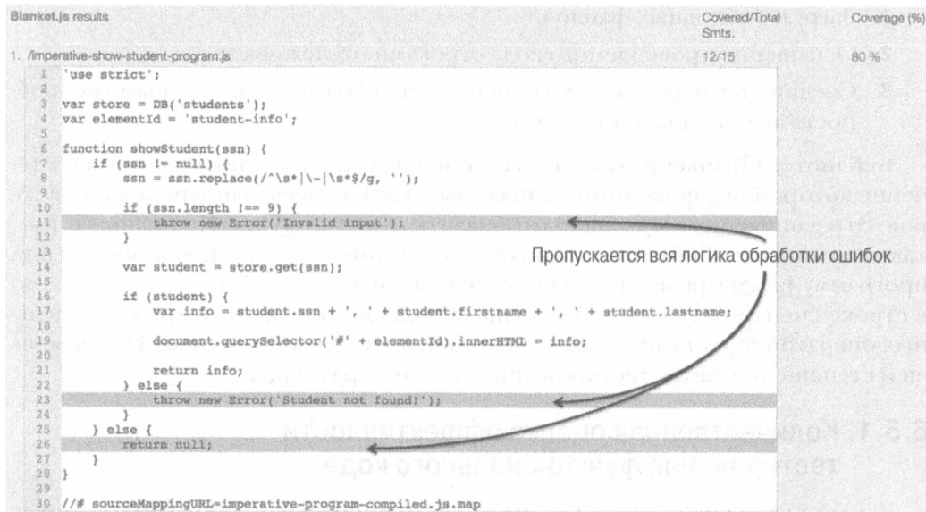
Рис. 6.10. Выводимый в QUnit/Blanket результат выполнения императивной версии программы showStudent с достоверными входными данными. В специально выделенных строках кода представлены операторы, которые вообще не были выполнены. В итоге из 15 строк кода было выполнено только 12, а следовательно, общее их покрытие тестами составило лишь 80%
