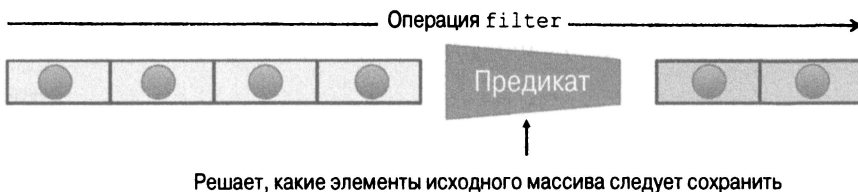
Рис. 3.6. Функции, реализующей операцию filter , передается в качестве параметра исходный массив данных и функция-итератор p ; она применяет к нему заданные в функции p критерии отбора, чтобы получить в итоге потенциально меньшее подмножество исходного массива. Критерии отбора p называются также предикатной функцией
