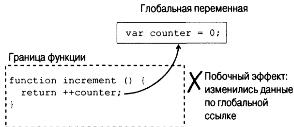
Рис. 1.1. Функция increment() вызывает побочные эффекты от чтения или модификации внешней переменной counter . Результат ее выполнения непредсказуем, поскольку переменная counter может измениться в любой момент в промежутках между вызовами данной функции
