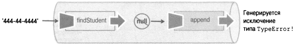
Рис. 5.10. Композиция функций findStudent() и append() . Если бы первая из них возвратила пустое значение null , то в отсутствие надлежащих проверок вторая функция завершилась бы неудачно, сгенерировав исключение типа TypeError
