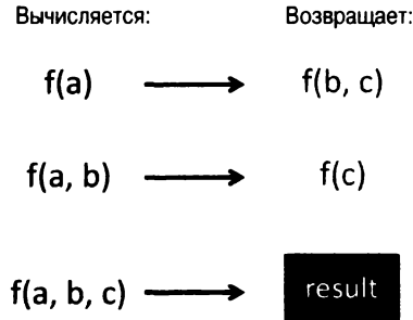
Рис. 4.6. Вычисление каррированной функции f . Эта функция выдает конкретный результат только в том случае, если ей переданы все аргументы. В противном случае она возвращает другую функцию, ожидающую получить остальные аргументы перед своим выполнением
