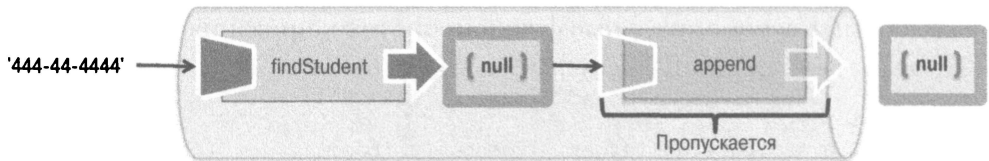
Рис. 5.11. Те же самые функции, что и на рис. 5.10, но на этот раз пустое значение null передается по конвейеру в монаде ( Either или Maybe ). В итоге остальные функции в конвейере корректно выходят из сбойной ситуации
