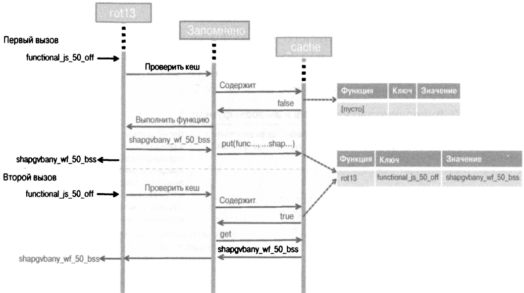
Рис. 7.7. Подробное представление двух вызовов функции rot13() с сообщением "functional_js_50_off". В первый раз, когда кеш еще пуст, предоставляемый код скидки преобразуется по алгоритму ROT13. Полученный результат далее сохраняется во внутреннем кеше по ключу из этих входных данных. А во второй раз происходит попадание в кеш, в результате чего из него сразу же возвращается значение без повторного вычисления хеш-значения
