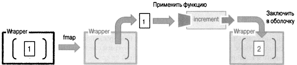
Рис. 5.3. Значение 1 содержится в объекте-оболочке типа Wrapper . Функтор вызывается с оболочкой и функцией increment() , преобразующей значение внутренним образом и снова заключающей его в оболочку
