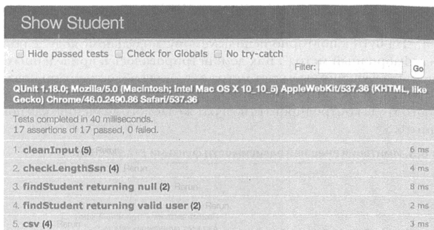
Рис. 6.7. Результаты выполнения всех модульных тестов программы showStudent . Тесты 3 и 4 проведены средствами QUnit и Sinon.JS, и поэтому для них требуются имитируемые зависимости, чтобы смоделировать функциональные возможности для извлечения записи об учащемся
