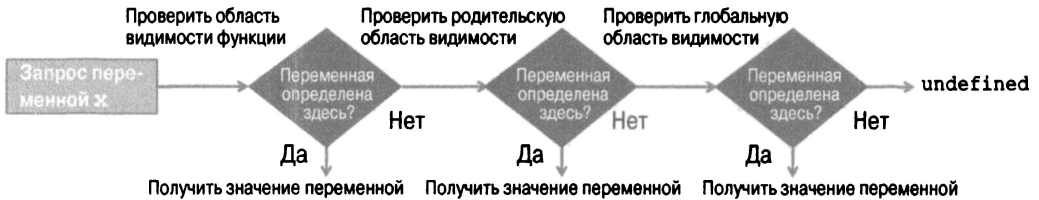
Рис. 2.5. Порядок разрешения имен, принятый в JavaScript. Сначала поиск значения переменной x производится в ближайшей, окружающей ее области видимости, а затем продолжается наружу. При этом сначала проверяется область видимости функции (т.е. локальная область видимости), затем происходит переход к родительской области видимости, если таковая существует, и, наконец, — к глобальной области видимости. Если переменная x не найдена, функция возвратит неопределенное значение undefined
