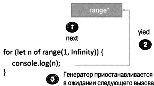
Рис. 8.10. Выполнение генератора range в цикле for...of . На каждом шаге цикла генератор будет приостанавливать свое выполнение и выдавать новые данные. Следовательно, семантически генераторы подобны итераторам
