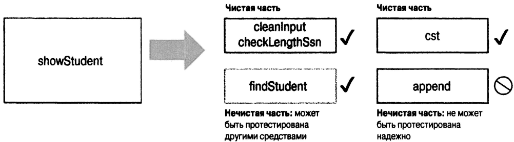
Рис. 6.6. Выяснение тестируемых участков в программе на основе функции showStudent() . Те ее компоненты, которые выполняют операции ввода-вывода, не могут быть протестированы надежно, поскольку они содержат побочные эффекты. Если не принимать во внимание нечистые части программы, то вся она вполне поддается тестированию
