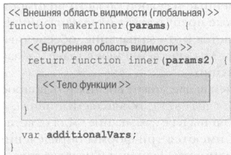
Рис. 2.4. Замыкание включает в себя переменные, находящиеся во внешней (глобальной) области видимости, внутренней области видимости родительской функции, а также параметры родительской функции и дополнительные переменные, объявленные после объявления функции. В коде, образующем тело функции, могут быть доступны переменные и объекты, определенные в каждой из этих областей видимости. Все функции разделяют общую глобальную область видимости
