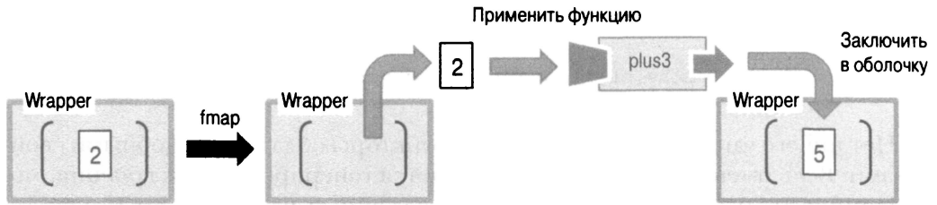
Рис. 5.4. Значение 2 прибавляется к значению в объекте-оболочке типа Wrapper . А функтор служит для манипулирования этим значением, извлекая его из контекста оболочки, применяя к нему заданную функцию преобразования и снова закладывая его в контекст, но уже новой оболочки
