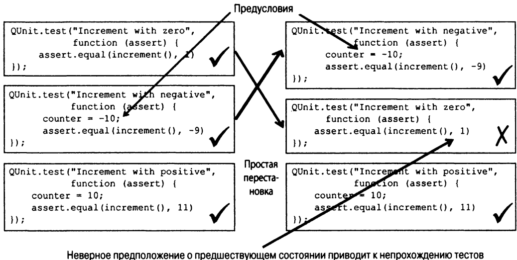
Рис. 6.4. Ложное предположение о глобальном состоянии системы приводит к тому, что даже простой тест не проходит. Как показано на рисунке слева , все тесты выполняются идеально, поскольку перед выполнением каждого из них соответственно подготовлено окружающее его состояние. Но стоит изменить порядок выполнения тестов ( справа ), и все предположения об окружающем их состоянии будут нарушены
