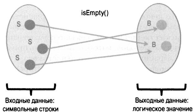
Рис. 4.2. Функция isEmpty() служит для ссылочно-прозрачного преобразования всех строковых значений в логические значения
