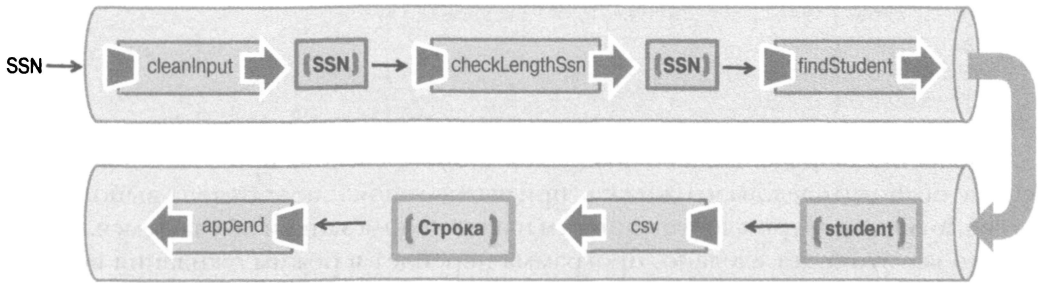
Рис. 5.12. Поэтапный поток выполнения программы showStudent в том случае, если функция findStudent() успешно найдет объект, представляющий учащегося, по заданному номеру социального страхования (SSN)
