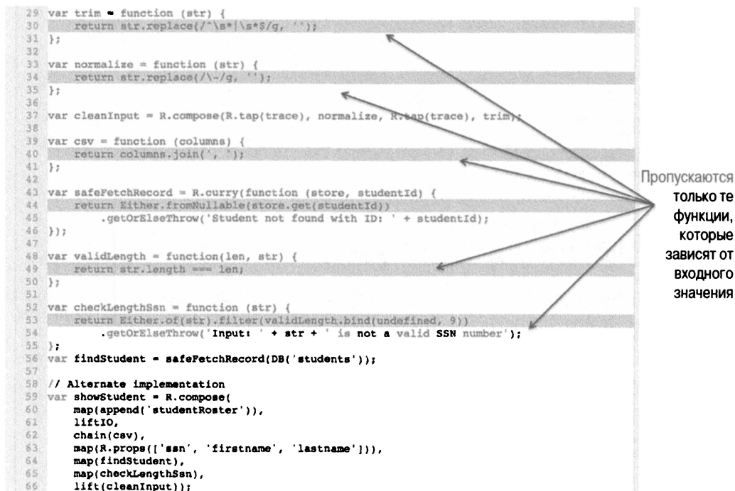
Рис. 6.13. При тестировании функциональной версии программы showStudent пропускаются строки кода, связанные только с манипулированием входными данными, которые в противном случае происходили бы из достоверного источника
