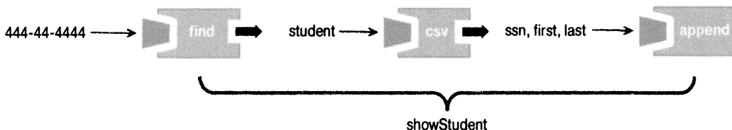
Рис. 1.4. Поток данных при композиции двух функций. Значение, возвращаемое из функции find() , должно быть совместимым по типу и аргументности (т.е. количеству аргументов) с функцией csv() , возвращающей, в свою очередь, информацию, которая может быть использована в функции append() . Обратите внимание на то, что порядок вызова этих функций был изменен на обратный, чтобы сделать более понятным поток данных
